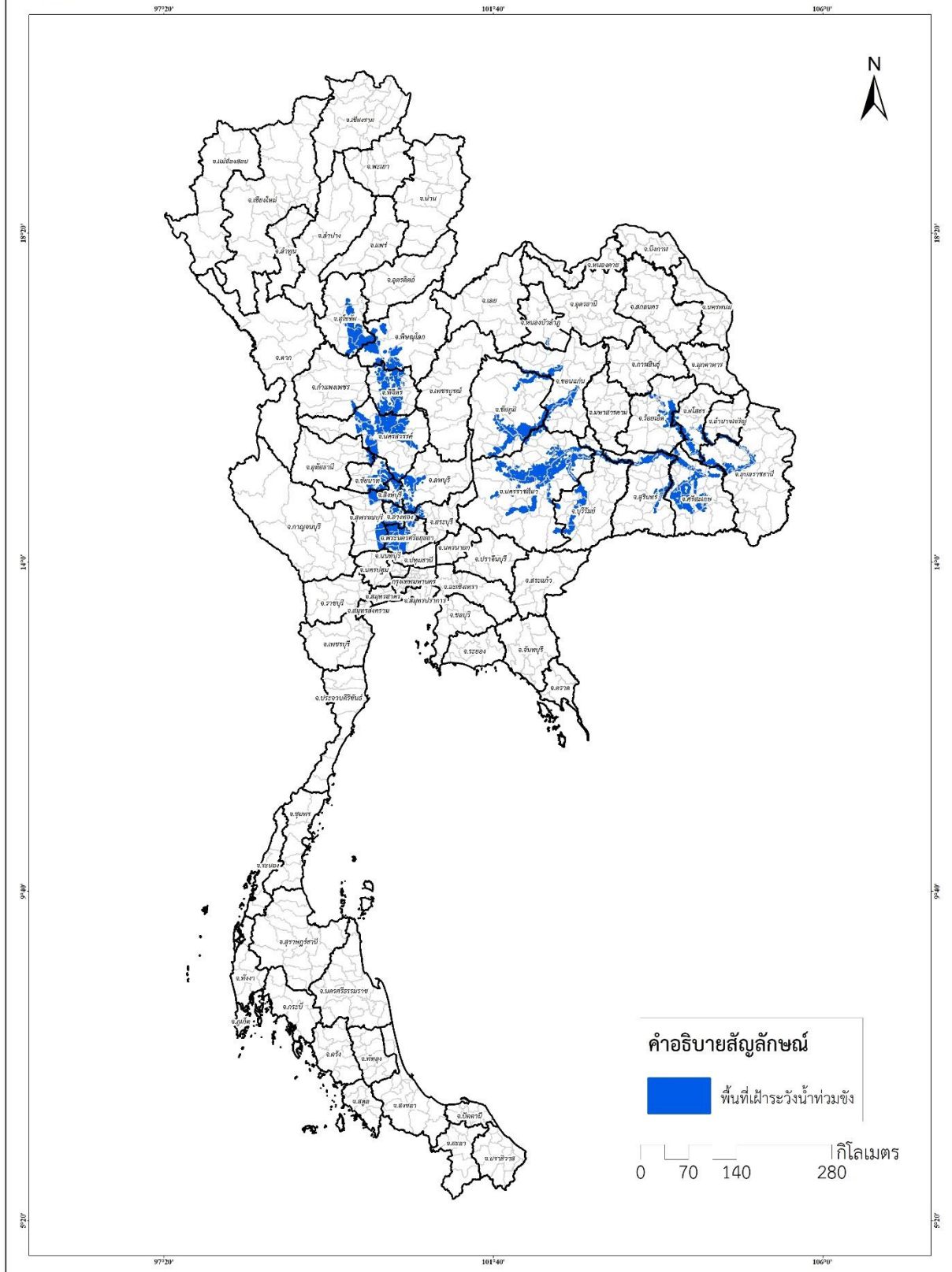
ภาพที่ 1 พื้นที่เฝ้าระวังน้ำท่วม (สีฟ้า) ที่ได้จากการวิเคราะห์และคาดการณ์จากฐานข้อมูลพื้นที่น้ำท่วมที่ได้จากการแปลจากภาพถ่ายดาวเทียม
